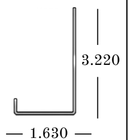
J - Stiffener
