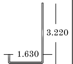
J - Stiffener
