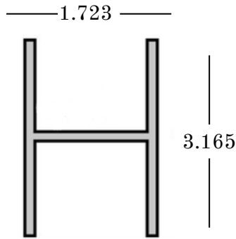
H - Stiffener
