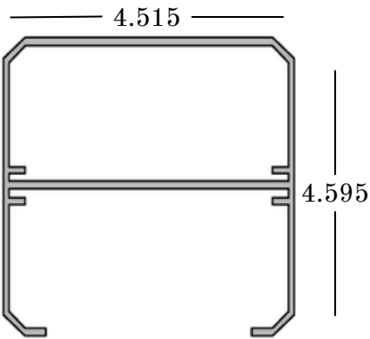
A Stiffener
