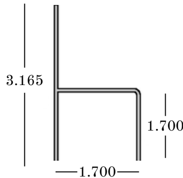
h - Stiffener
